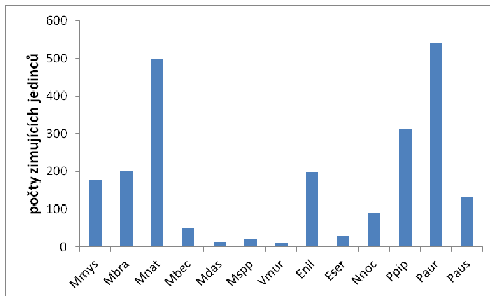
Graf 1 Počty jedinců u ostatních druhů netopýrů zjištěných na zimovištích
