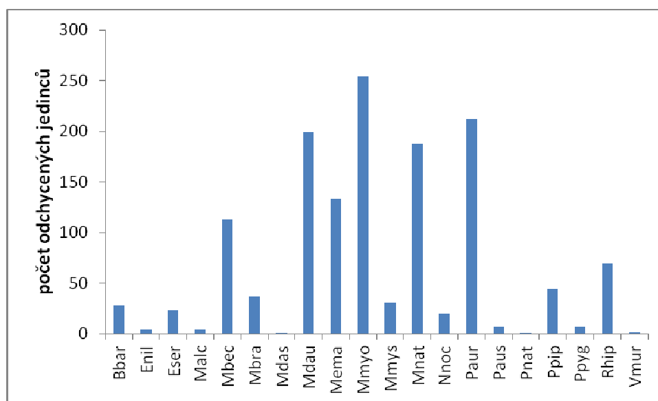
Graf 2 Počty odchycených jedinců netopýrů na všech monitorovaných lokalitách
